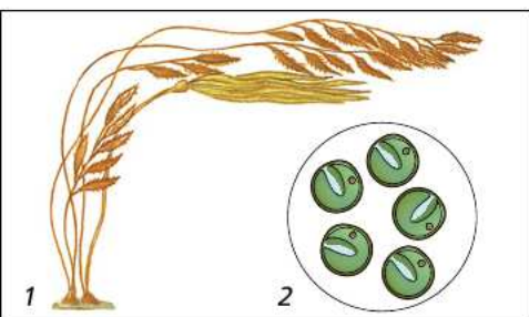
Рис. 107. Макроцистис (1), хлорелла (2)
