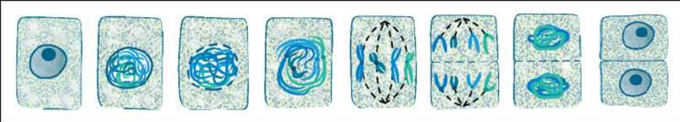
Рис. 19. Деление клетки
