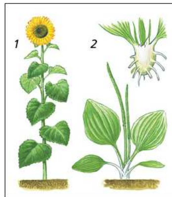
Рис. 61. Стебель:
