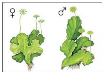
Рис. 112. Маршанция
